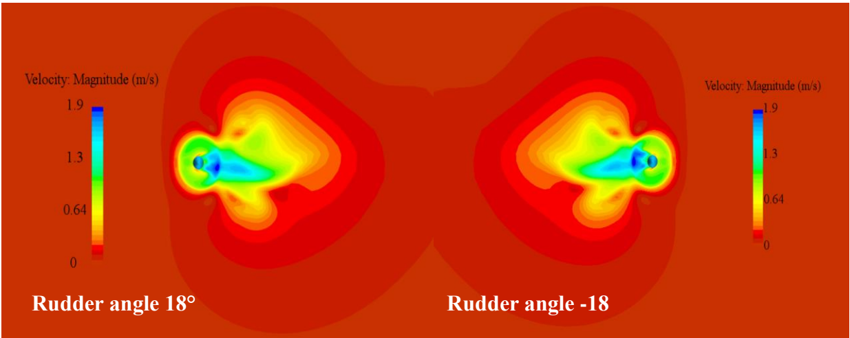
(c) Rudder angle -18^\circ/18^\circ
